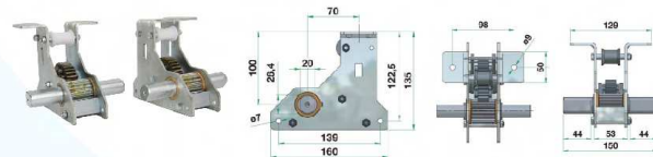
拉幕齿轮 A型 Screening pinion A type 行程 Stroke: 79mm 速比 Speed ratio: 1.8:1
