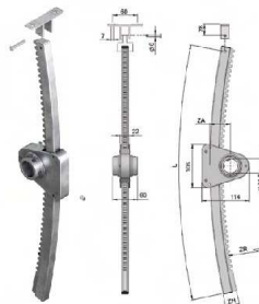
德国LOCK连续开窗齿轮齿条(弧型)
