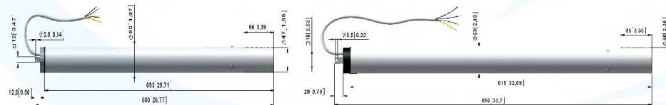
德国LOCK管式电机零配件
