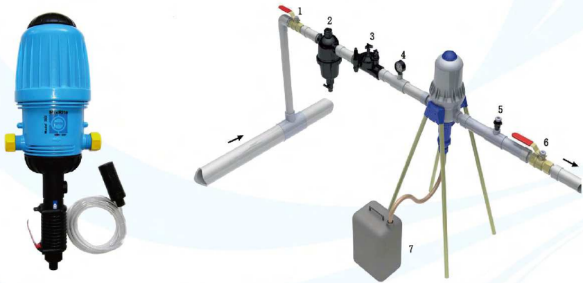
比例施肥泵
