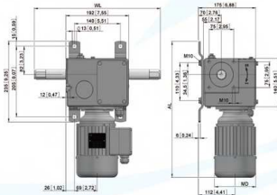
EWA14电机安装尺寸图
