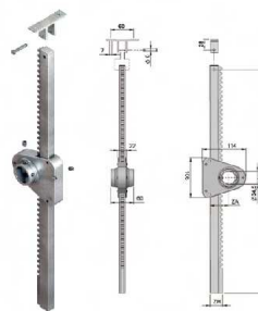
德国LOCK连续开窗齿轮齿条(直型)
